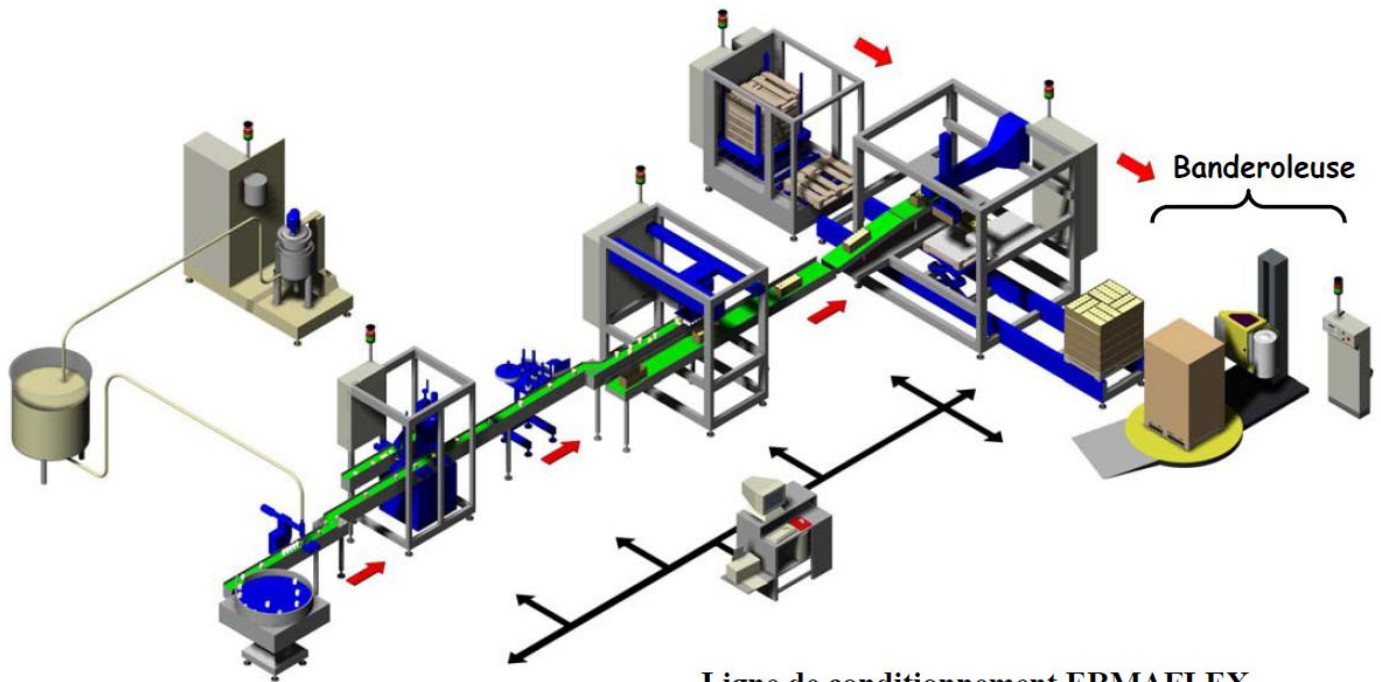
Ligne de conditionnement ERMAFLEX
